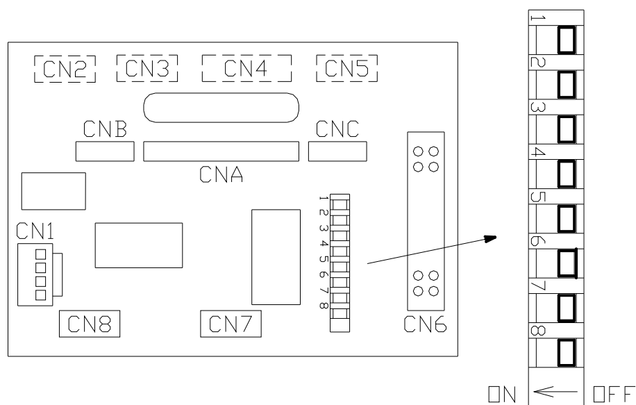
ディップスイッチ詳細図
