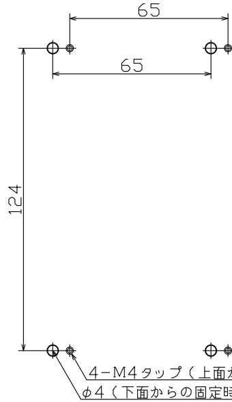
取付参考図
