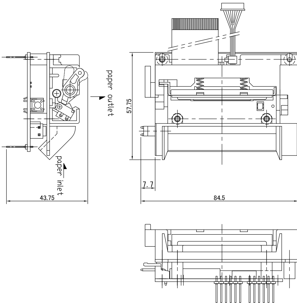
AS-289R プリンタ シールド基板+メカユニット
